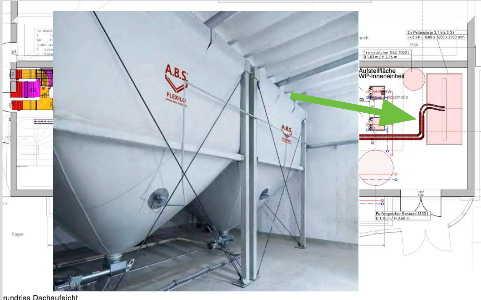
rundriss Dachaufsicht
