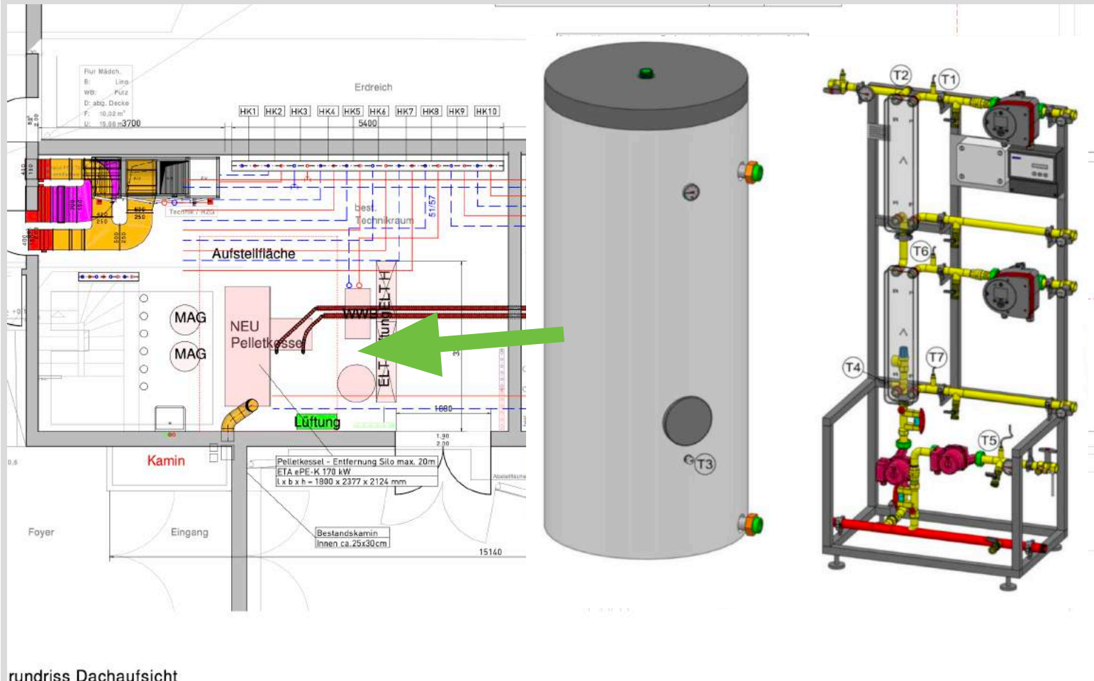
rundriss Dachaufsicht
